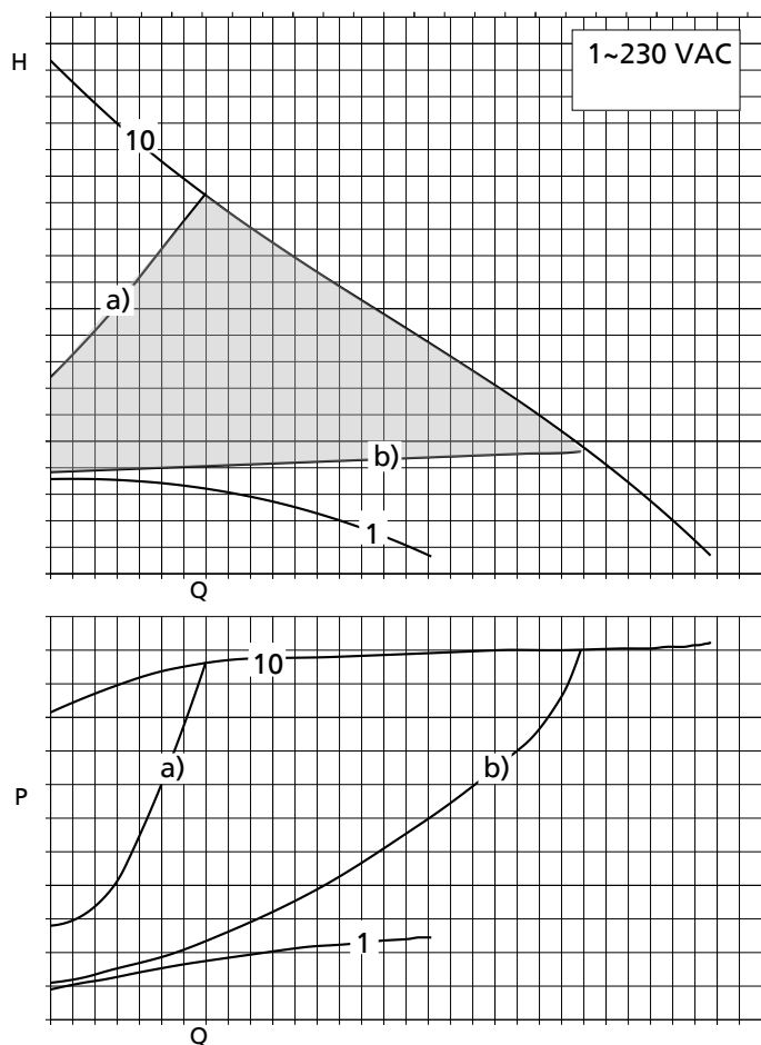
Abb. 2: Auslegungsbeispiel
