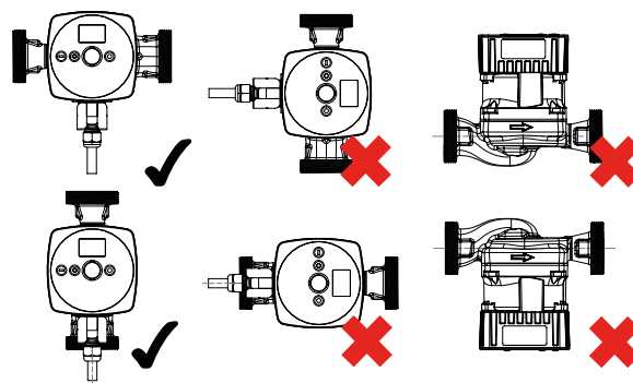
Abb. 8: Zulässige Einbaulagen
