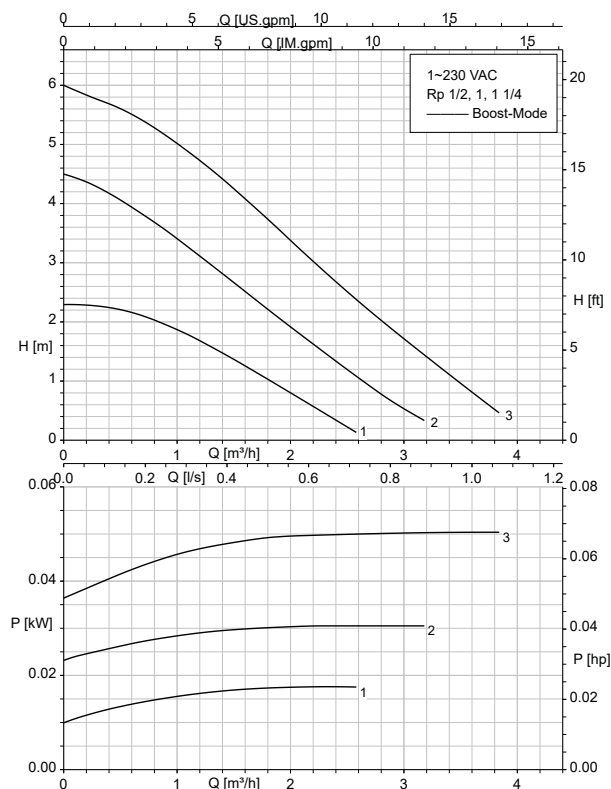
Abb. 4: 1, 2, 3 = Drehzahlstufe 1, 2, 3
