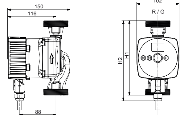
Abb. 6: Abmessungen Calio S [mm]
