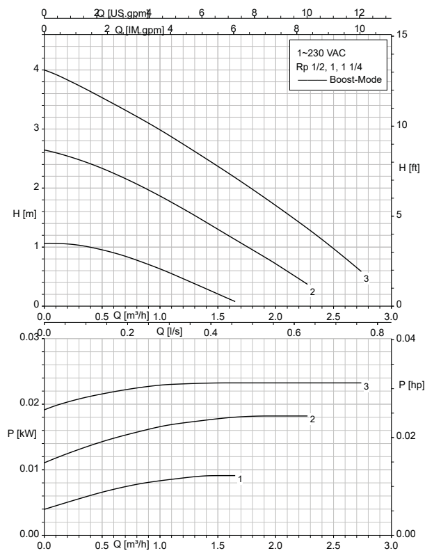
Abb. 3: 1, 2, 3 = Drehzahlstufe 1, 2, 3
